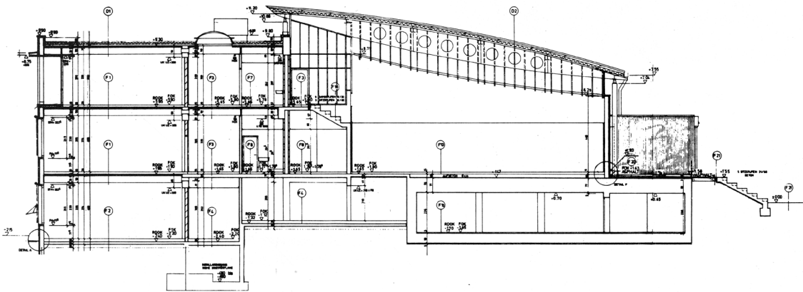
Schnitt
