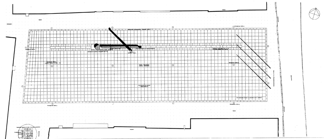
Grundriss
