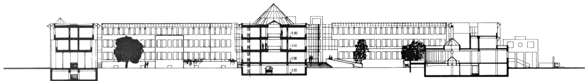
SCHNITT B-B
