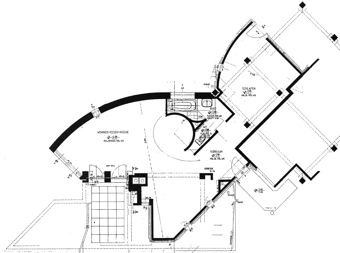
Grundriss
