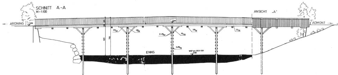
Schnitt
