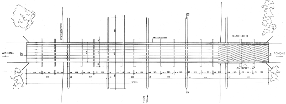
Grundriss
