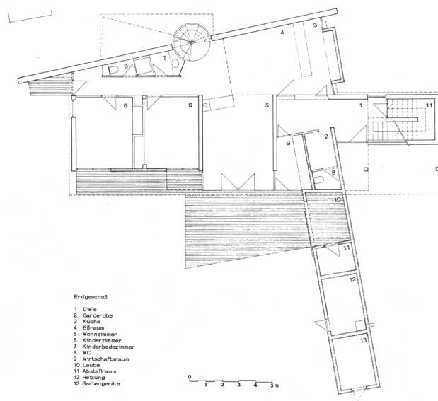
Grundriss Erdgeschoss
