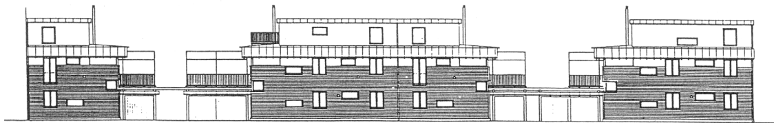
Fassadenabwicklung Nord-Ost
