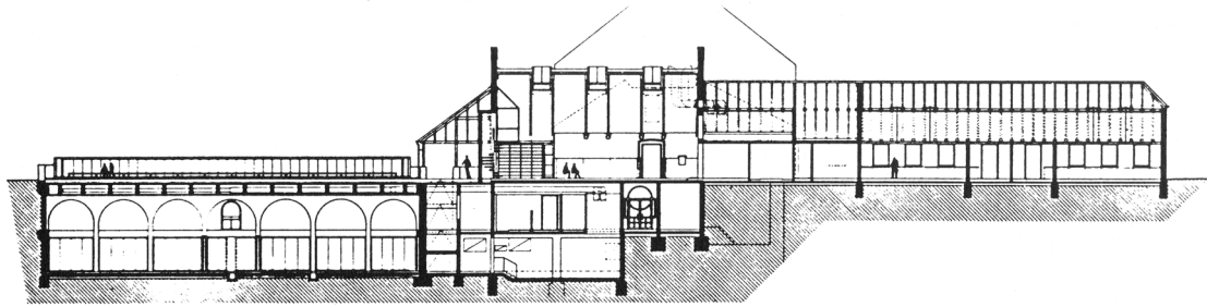
Schnitt
