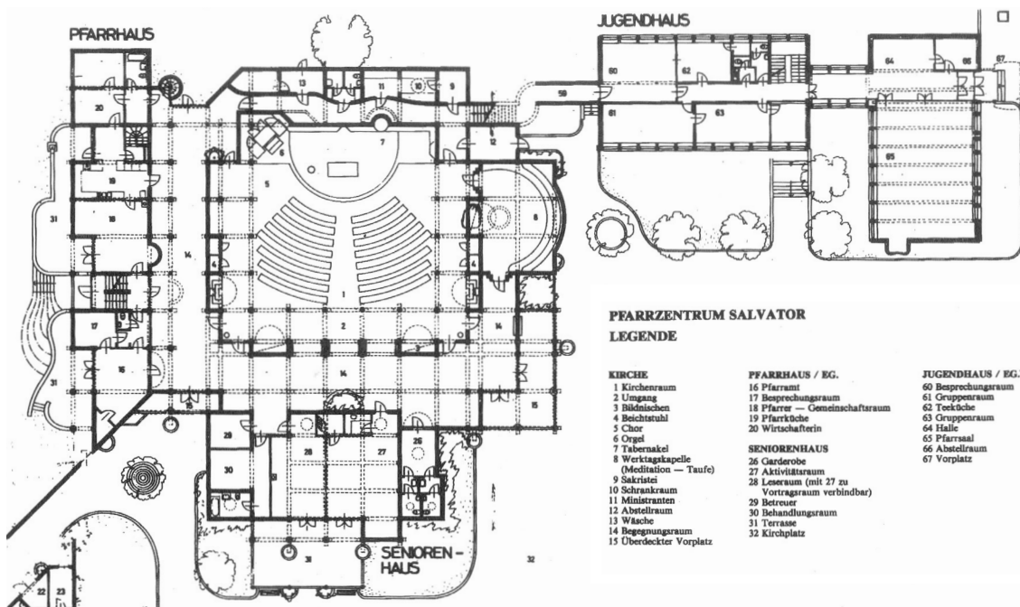
Grundriss
