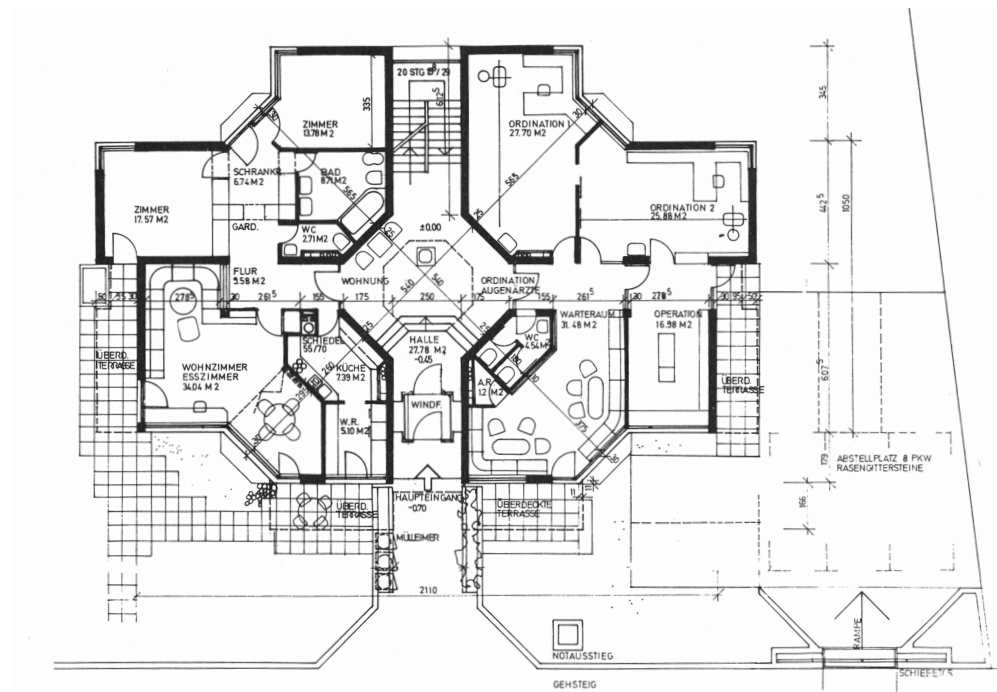
Grundriss
