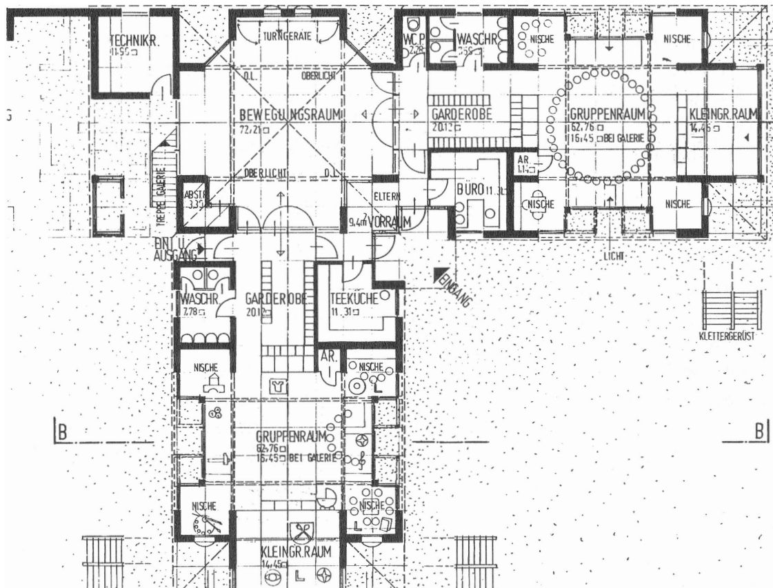
Grundriss
