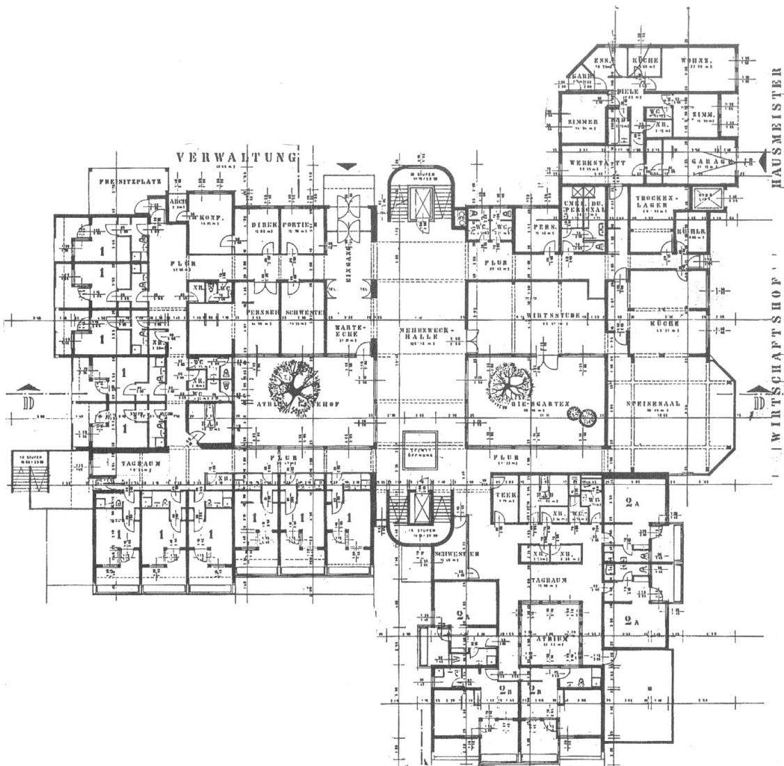
Grundriss
