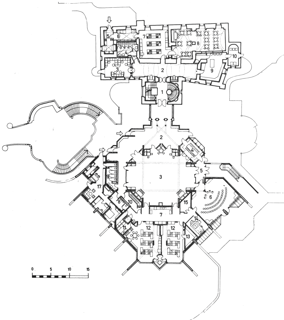
Grundriss Erdgeschoss
