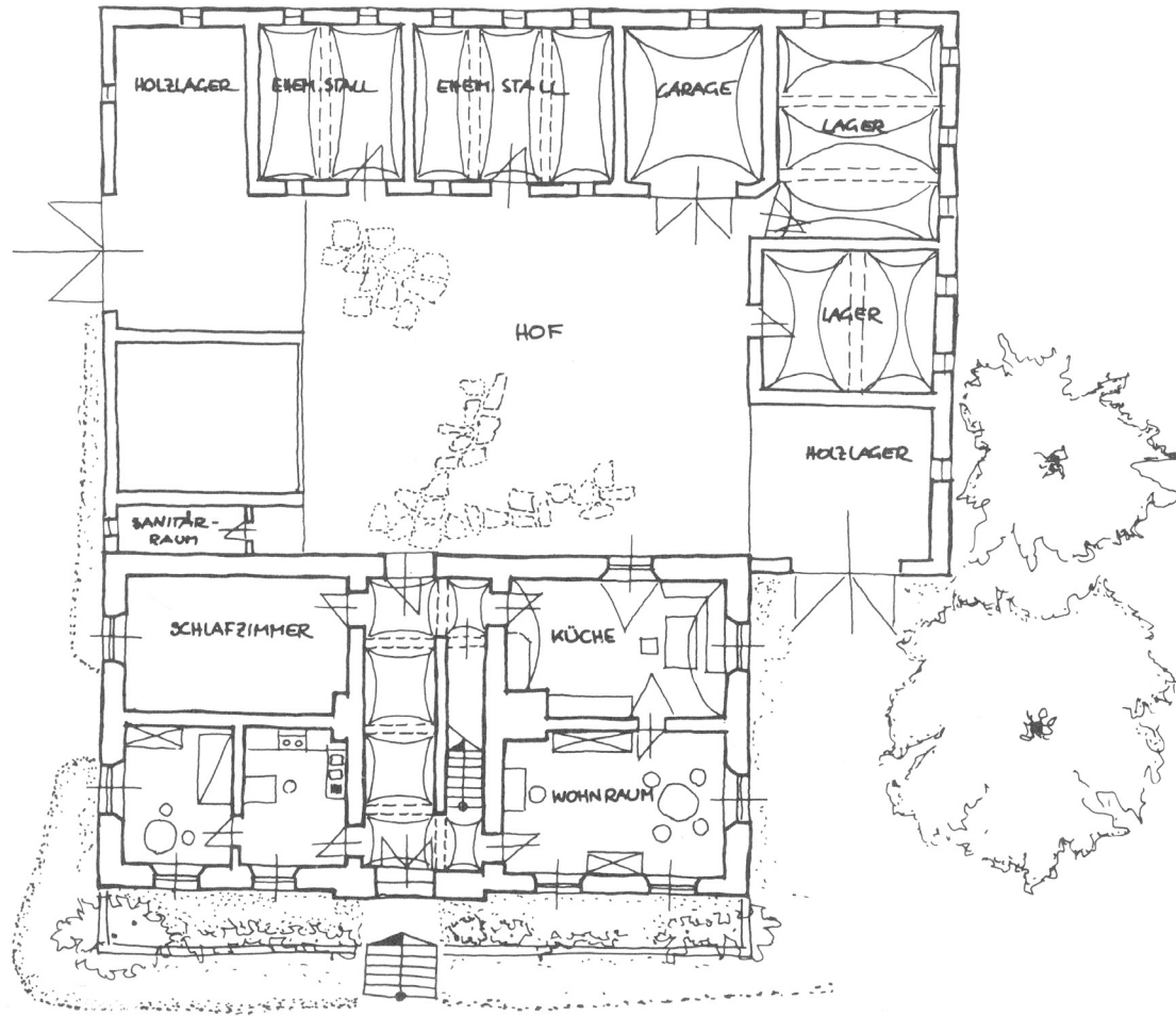
Grundriss
