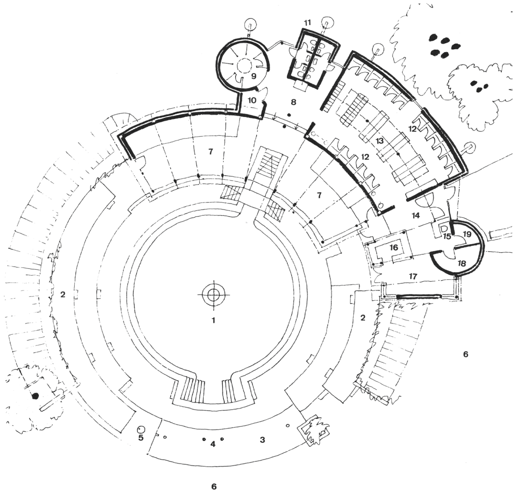
Grundriss
